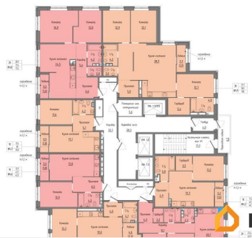
План 08 этажа
