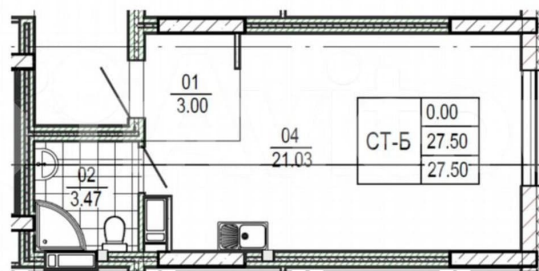
Экспликация помещения
