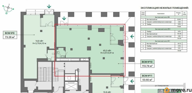
ДОМ 1.4, 1 ЭТАЖ
